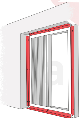
Montáž siete na profily (pohľad zo zadu)
